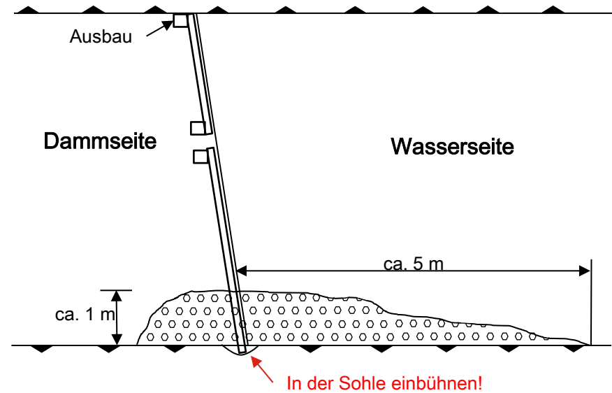
Holzfünger Seitenansicht:
